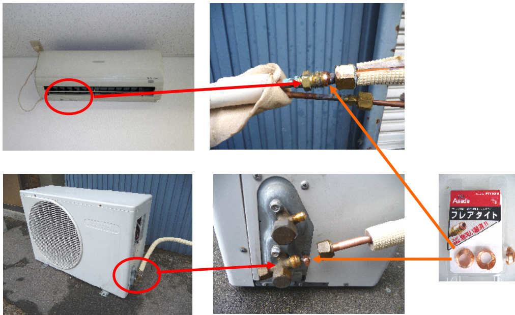
エアコン室内機、室外機接続個所 漏れ止め部材使用状況
