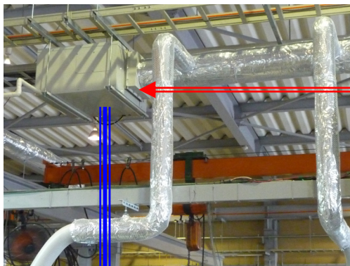
工場内熱交換器
